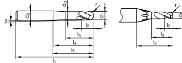
mit GühroJet Peripheriekühlung von Ø 0,2-3 mm
